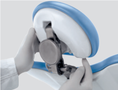
Atlaxis Подголовник, повторяющий анатомию пациента. Сверхлегкое нажатие на пневматический фиксатор позволяет совершать круговые движения для достижения идеального позиционирования, включая вертикальную регулировку.
